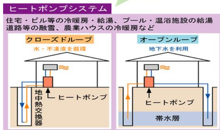
地中熱を利用したヒートポンプシステムイメージ
